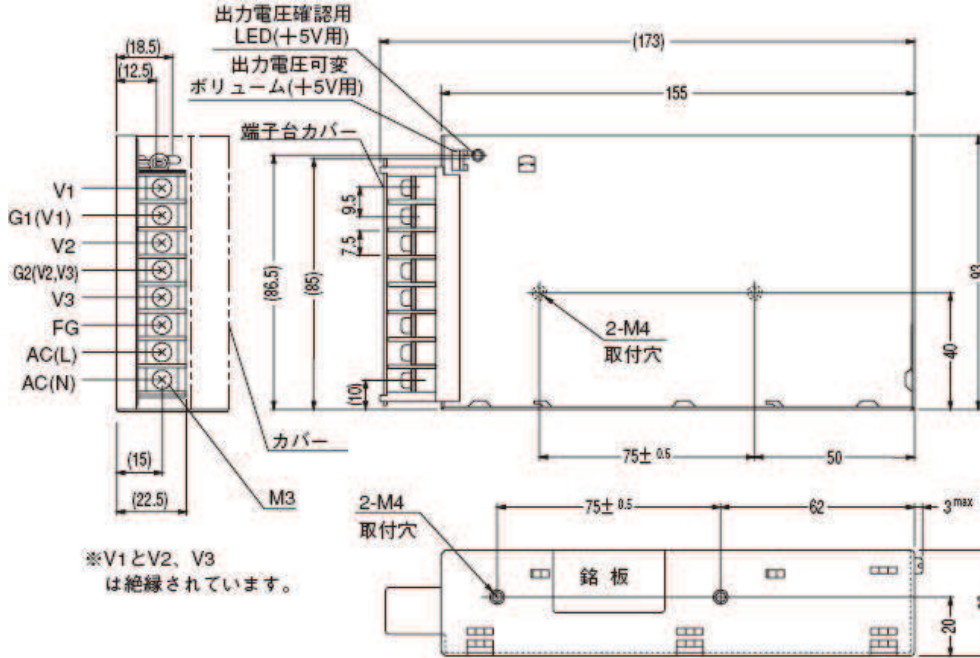
【MMC50A外形図】
