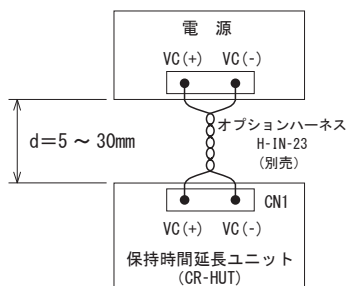
図3.3 接続方法
