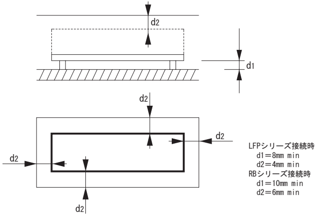
図3.1 取付方法
