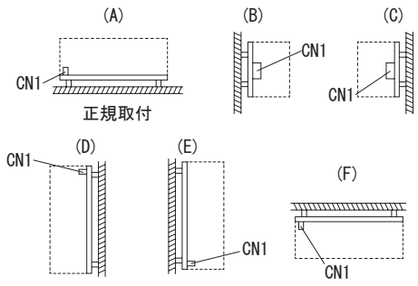
図3.4 CR-HUT □ -1 取付方法
