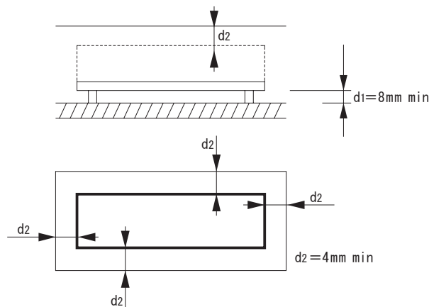
図3.1 取付方法
