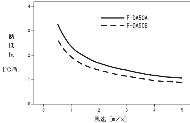
図1 F-DA50A、F-DA50B ヒートシンク熱抵抗
