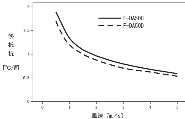
図2 F-DA50C、F-DA50D ヒートシンク熱抵抗
