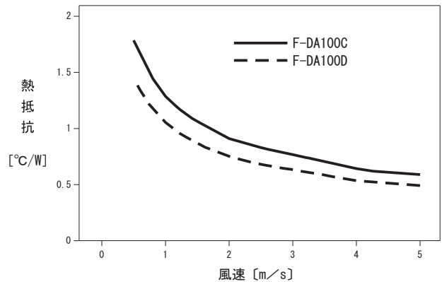
図4 F-DA100C、F-DA100D ヒートシンク熱抵抗
