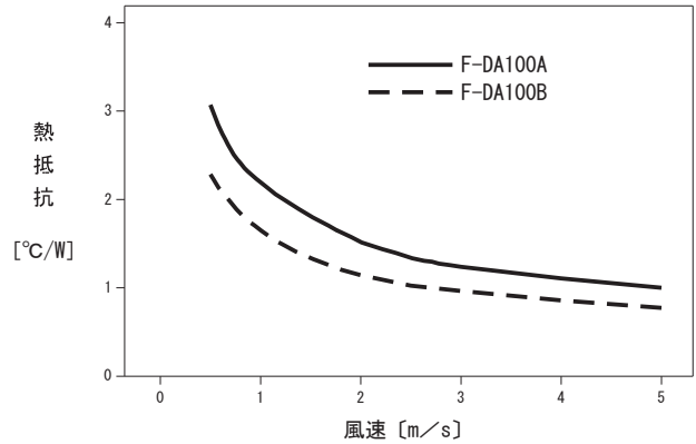
図3 F-DA100A、F-DA100B ヒートシンク熱抵抗
