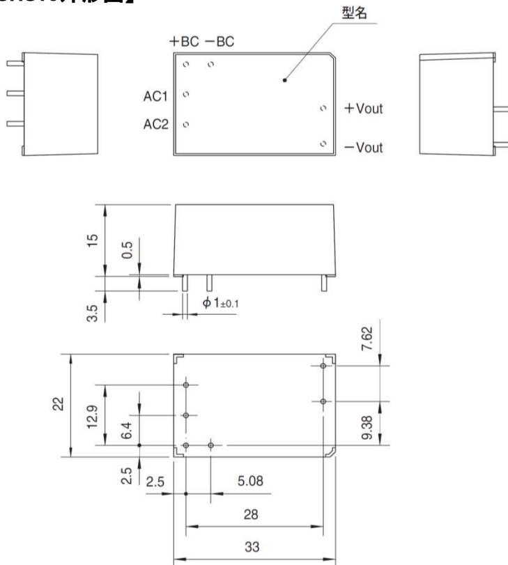
【TUHS10外形図】
