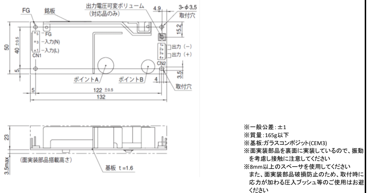
【LFA50F外形図】
