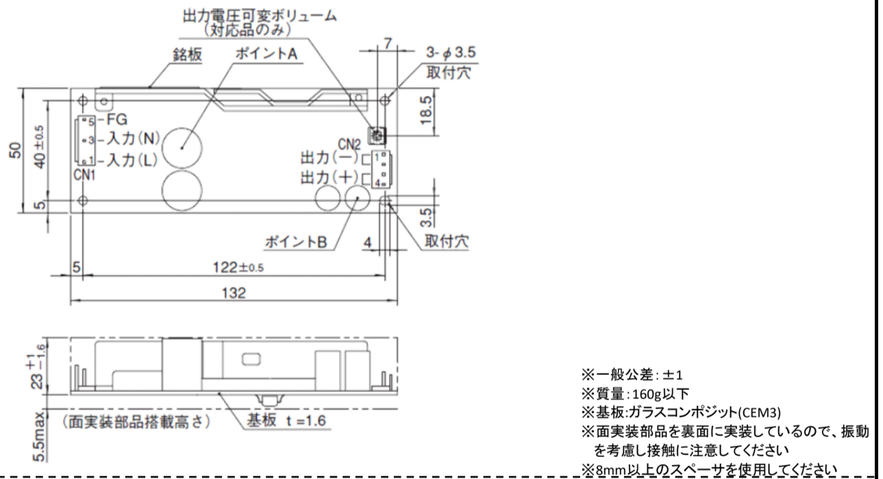
【LGA50A外形図】
