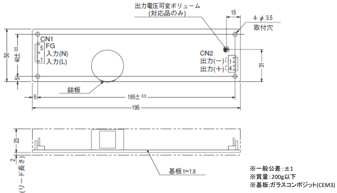
【LCA50S外形図】
