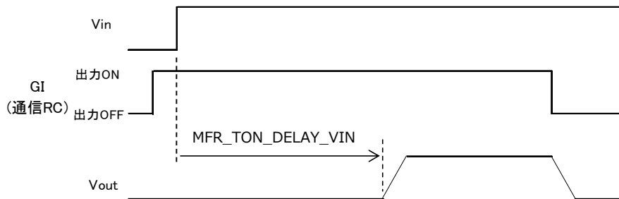
図6.5.3 MFR_TON_DELAY_VIN による起動遅延
