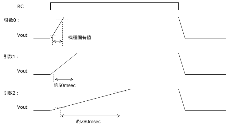
図6.5.5 MFR_RAMP_RATE 引数別 RC端子による起動
