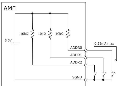
図2.5 アドレス設定方法
