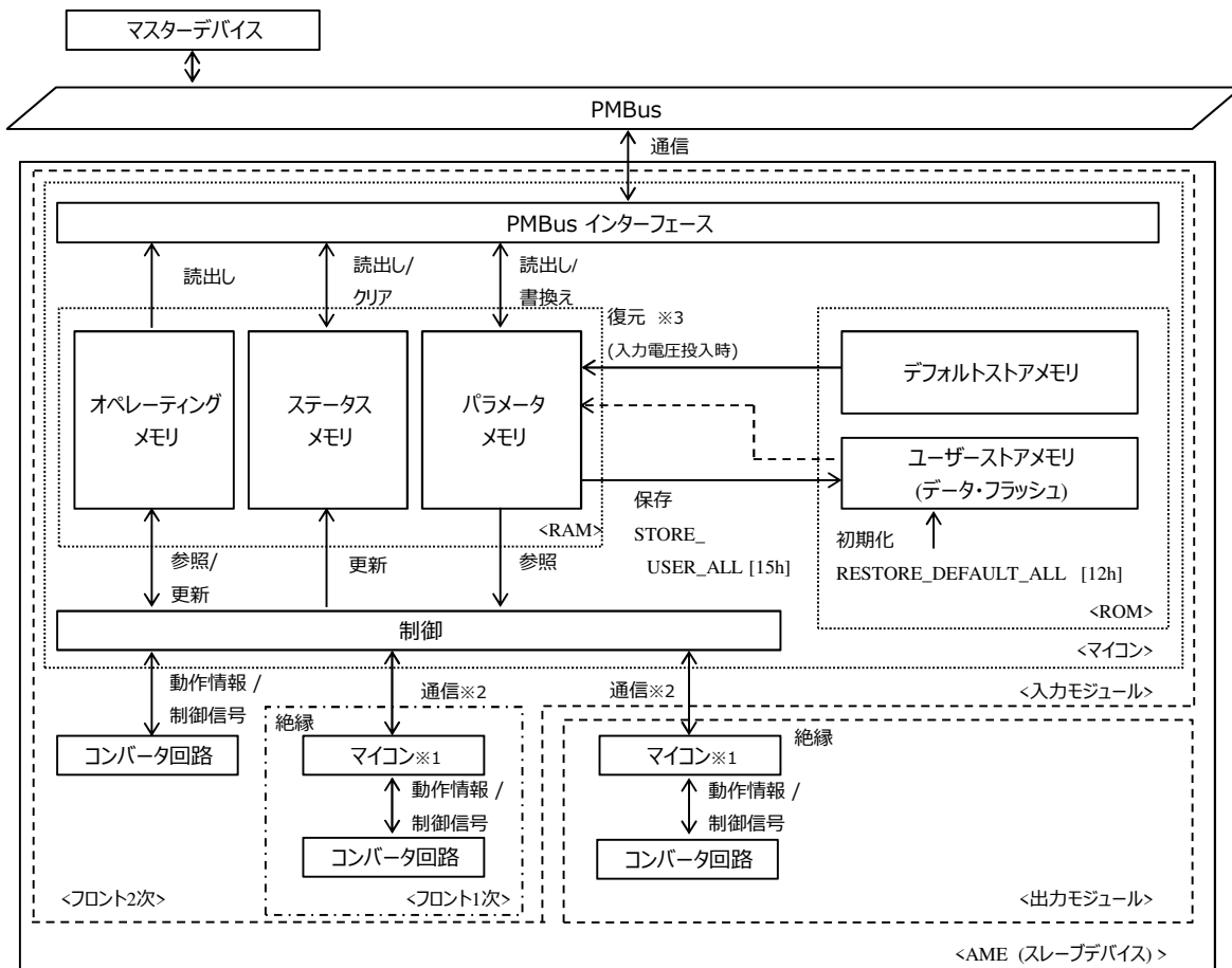
図4.1 PMBus通信 ブロックダイアグラム
