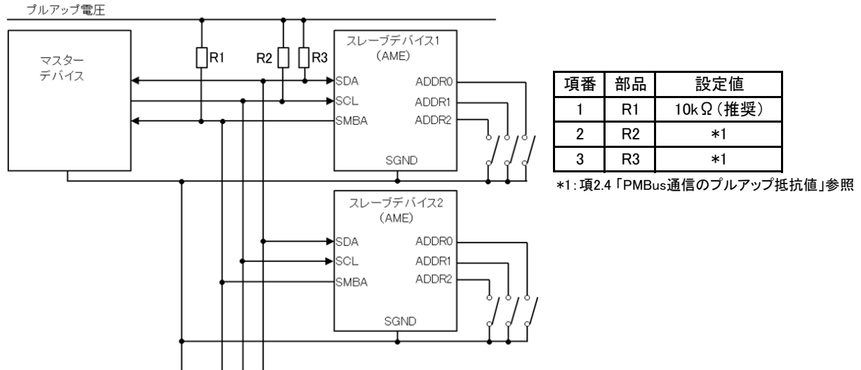
図2.2 PMBus接続例
