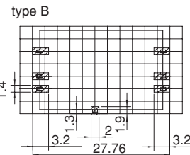
※プリント基板推奨加工寸法 (TOP VIEW)
