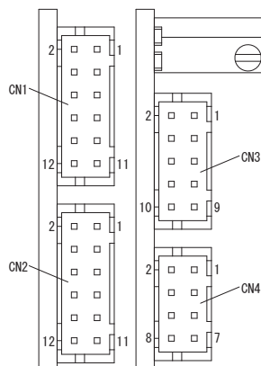
コネクタピン番号
