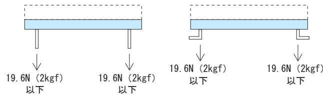
MU入出力ピン強度
