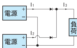
図4.2 冗長運転例
