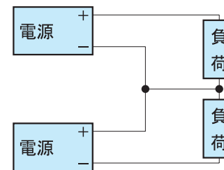
図4.1 直列運転例
