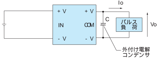
図 10.1 パルス負荷接続図
