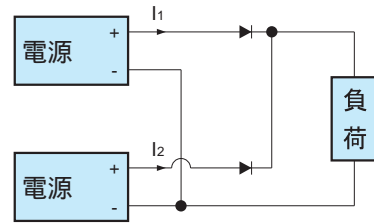
図 4.2 冗長運転例
