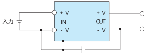
図 3.4 コモンモードノイズ低減回路
