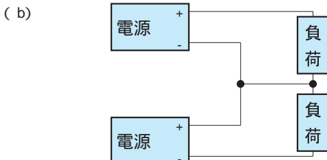
図 4.1 直列運転例
