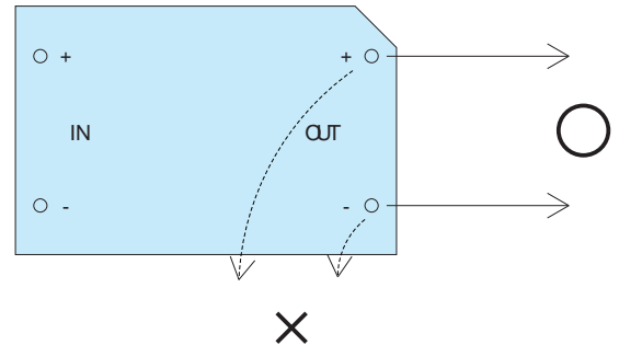
図 5.1 パターン配線
