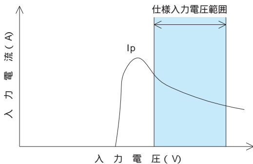
図 6.2 入力電流特性 (ZS1Q ZM0)
