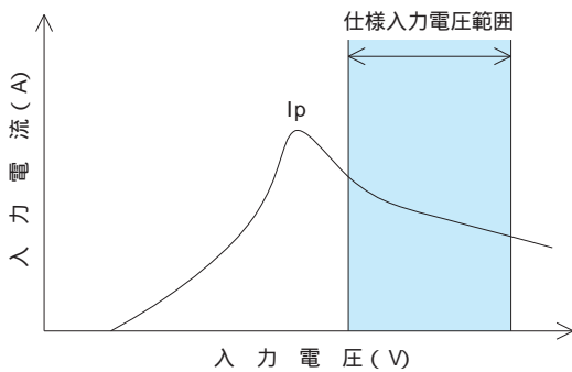
図 6.1 入力電流特性 (ZS1Q ZM0以外)
