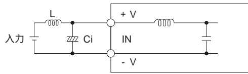
図 3.1 入力端コンデンサの接続方法
