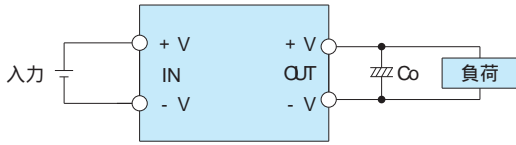
図 3.2 出力端コンデンサの接続方法
