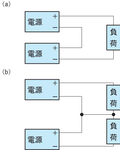
図4.1 直列運転例
