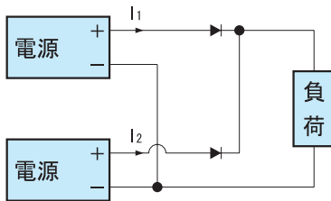
図4.2 冗長運転例
