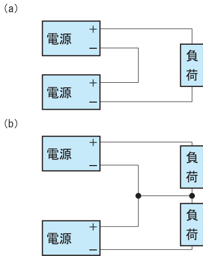
図4.1 直列運転例
