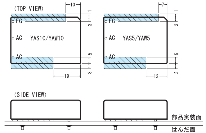
斜線部はパターン配置禁止領域 図5.2 パターン配置禁止領域
