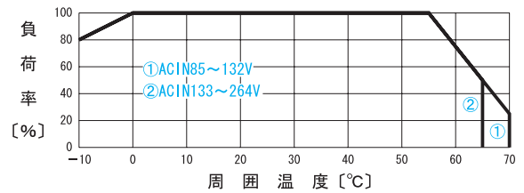
図5.3 ディレーティング特性
