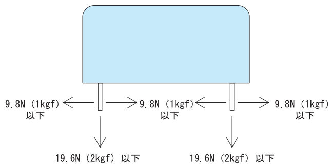
図8.1 ピンに加わる応力
