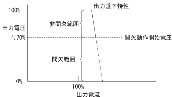
図2.1 出力垂下特性
