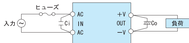
図3.1 出力端子外付けコンデンサ
