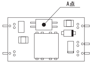
図8. 3 強制通風時の温度測定箇所
