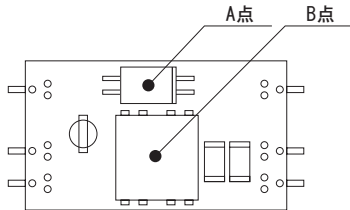
図7.3 強制通風時の温度測定箇所
