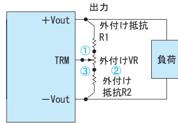
図1.2 外付け部品の接続方法
