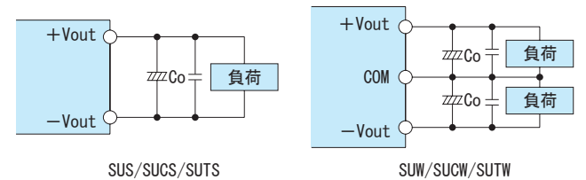
図2.3 出力側外付けコンデンサ接続方法
