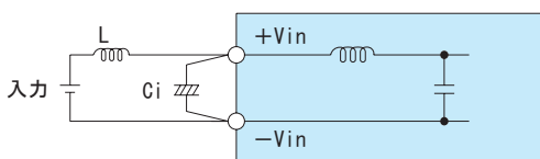
図2.1 入力側外付けコンデンサ接続方法
