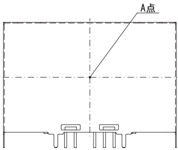
図7.11 強制通風時の温度測定箇所 (ケース印字面)
