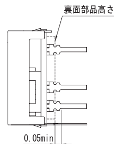
図11.1 ユーザ基板とのクリアランス (-C)
