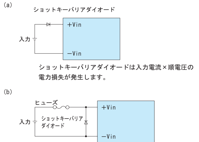
図2.2 逆接続保護方法
