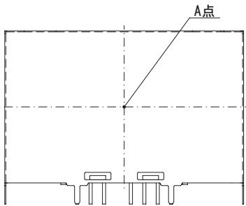
図7.11 強制通風時の温度測定箇所（ケース印字面）
