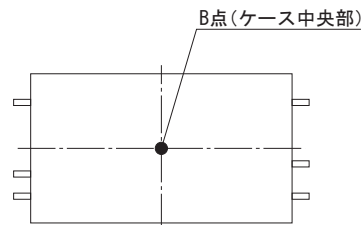
図7.8 強制通風時の温度測定箇所（ケース上面）
