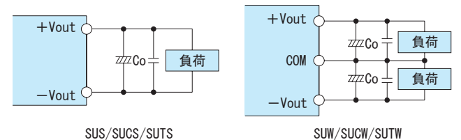
図2.3 出力側外付けコンデンサ接続方法
