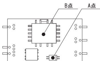
図7.5 強制通風時の温度測定箇所
