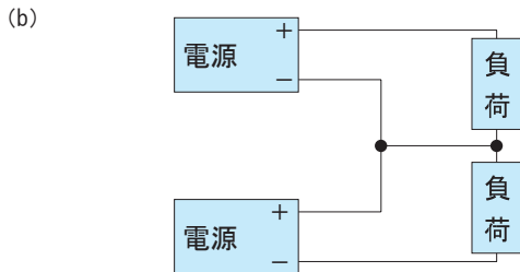
図3.1 直列運転
