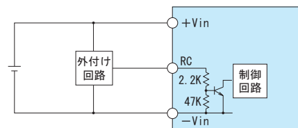
図1.3 リモートコントロール内部回路
