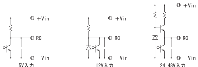
図1.4 リモートコントロール外付け回路使用例
