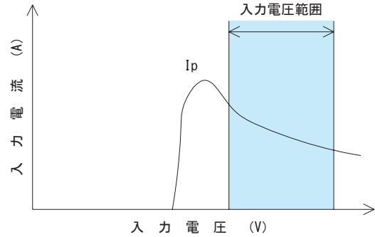
図5.1 入力電源
