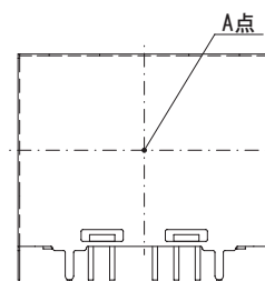
図7.9 強制通風時の温度測定箇所（ケース印字面）
