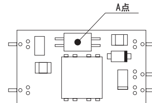
図7.1 強制通風時の温度測定箇所
