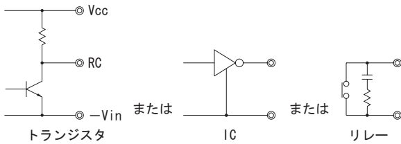
図1.5 リモートコントロールの使用例
