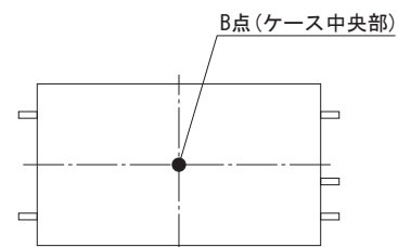
図7.2 強制通風時の温度測定箇所（ケース上面）
