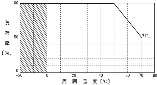
図 4.2 動作周囲温度によるディレーティング特性
