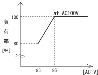
図 4.3 入力電圧によるディレーティング特性 (PBA1500F)
