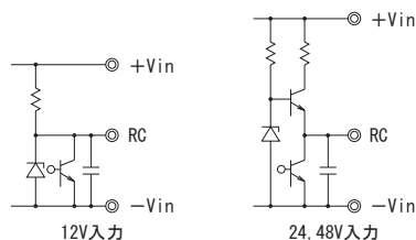
図1.2 リモートコントロール外付け回路例
