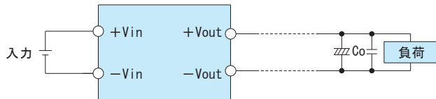
図2.4 接続方法
