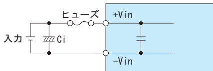
図2.1 入力側外付けコンデンサ接続方法
