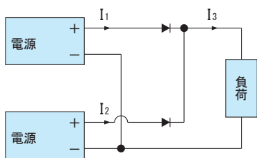
図3.2 冗長運転
