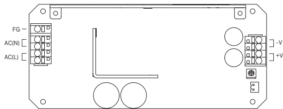
図7.5 T4仕様外形 (LHP150F)
