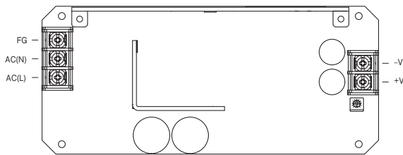
図7.10 T5仕様外形 (LHP150F)
