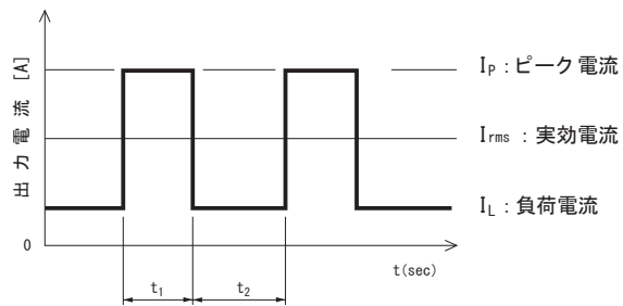
図6.1 ピーク電流での使用
