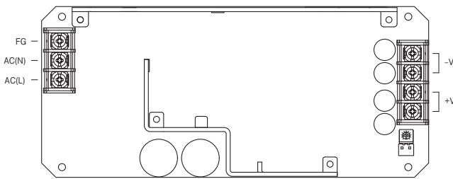
図7.4 T仕様外形 (LHP300F)
