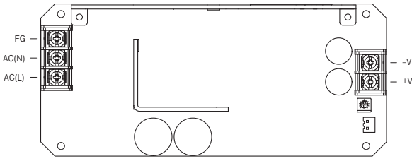
図7.3 T仕様外形 (LHP150F)
