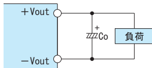
図7.17 出力側外付けコンデンサ接続方法
