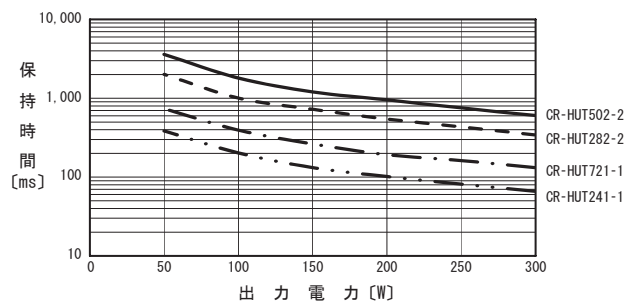
図7.16 LHP300F-U1Y 保持時間-出力電力特性 (参考値)
