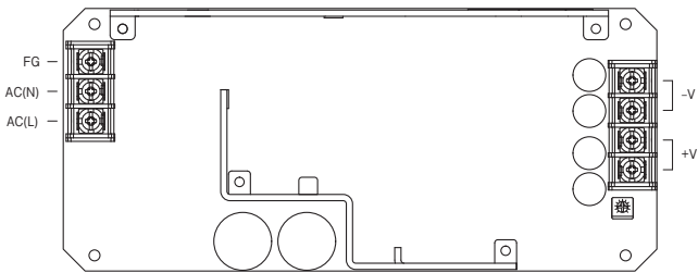
図7.11 T5仕様外形 (LHP300F)
