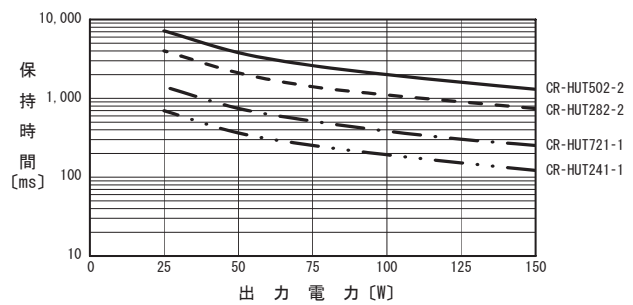
図7.15 LHP150F-U1Y 保持時間-出力電力特性 (参考値)
