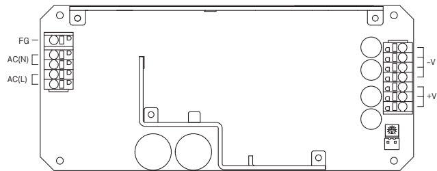
図7.6 T4仕様外形 (LHP300F)
