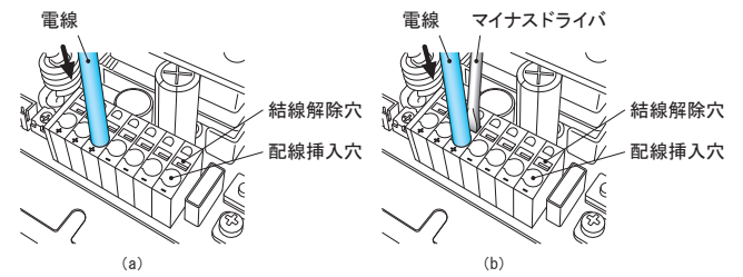
図7.7 フェルール端子、単線の結線概略図
