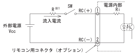
図7.2 リモートコントロール使用例
