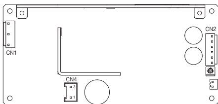
図7.12 CN4位置 (LHP150F-U1Y)
