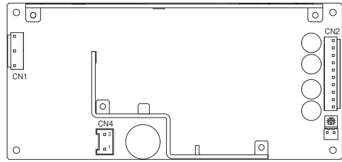
図7.13 CN4位置 (LHP300F-U1Y)
