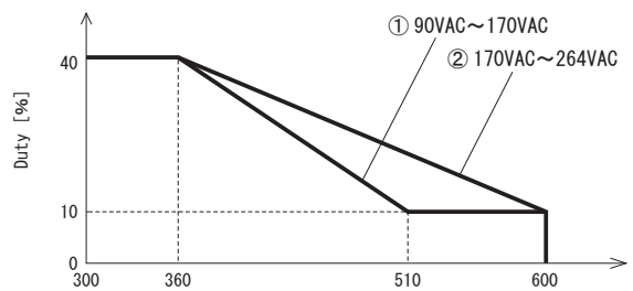
ピーク電力 [W] LHP300F
