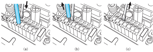
図7.9 フェルール端子、単線、撚線の解除概略図
