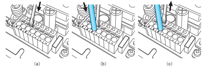
図7.8 撚線の結線概略図
