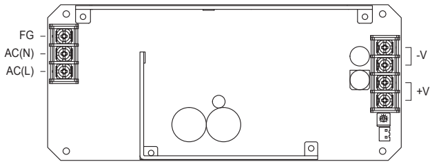
図6.3 T仕様外形
