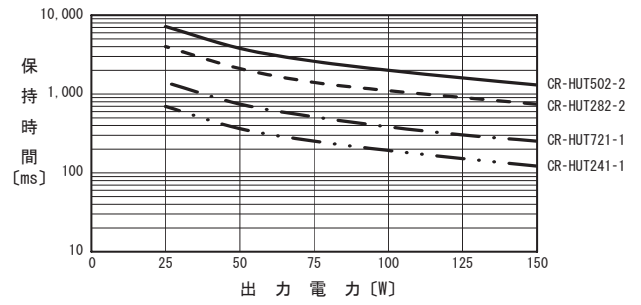
図6.11 LHA150F-□-U1 保持時間-出力電力特性 (参考値)
