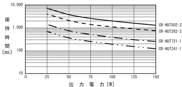
図6.7 LHA150F-□-U1 保持時間-出力電力特性 (参考値)
