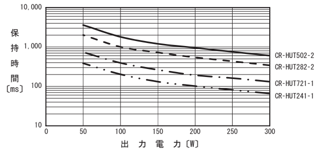
図6.12 LHA300F-□-U1Y 保持時間-出力電力特性 (参考値)
