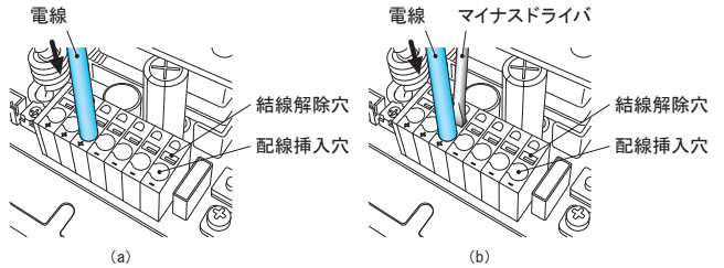
図6.5 フェルール端子、単線の結線概略図
