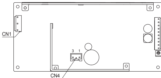
図6.9 CN4位置 (LHA300F-□-U1Y)
