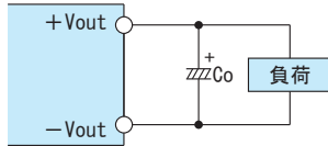
図6.9 出力側外付けコンデンサ接続方法
