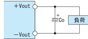
図6.13 出力側外付けコンデンサ接続方法
