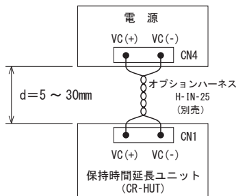
図6.10 接続方法
