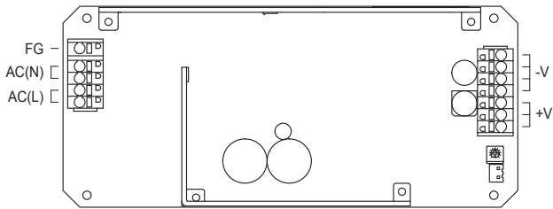
図6.4 T4仕様外形
