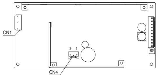
図6.5 CN4位置 (LHA300F-□-U1Y1)
