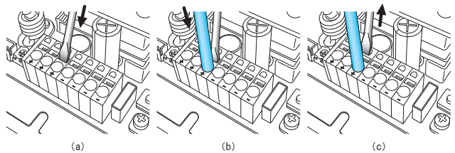
図6.6 撚線の結線概略図
