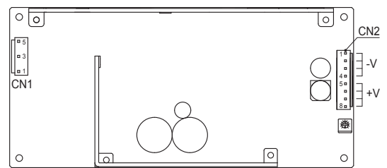
図6.1 J5仕様外形
