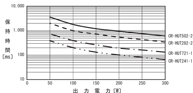
図6.8 LHA300F-□-U1Y 保持時間-出力電力特性 (参考値)
