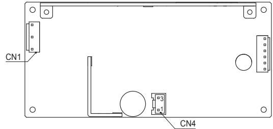
図6.4 CN4位置 (LHA150F-□-U1)
