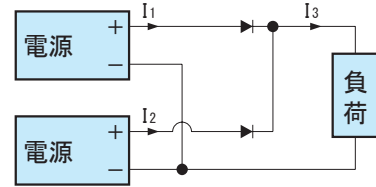
図2.2 冗長運転例
