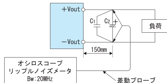
図1.1 出力リップル・リップルノイズ測定方法
