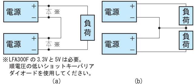
図2.3 直列運転時の接続例
