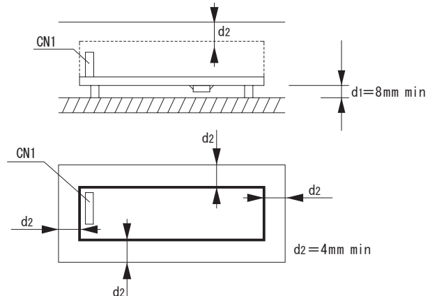
図3.1 取付方法
