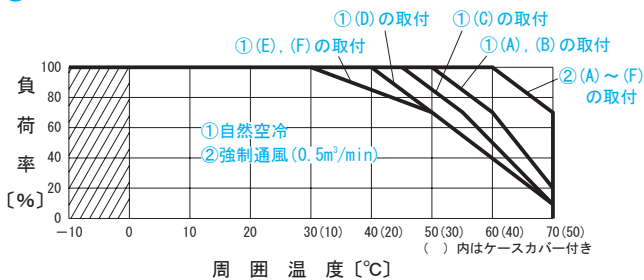
図3.7 動作周囲温度によるディレーティング (参考値)
