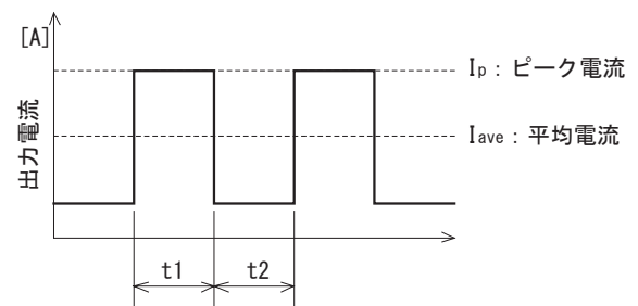
図5.1 ピーク電流での使用
