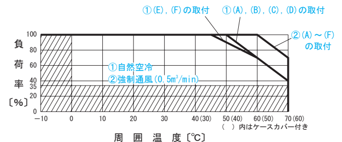
図3.4 動作周囲温度によるデレーティング（参考値）
