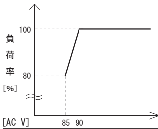
図3.17 入力電圧によるディレーティング
