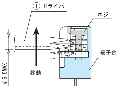
図5.4 ネジ持ち上げ方法
