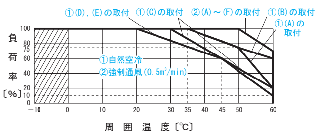
図3.9 動作周囲温度によるディレーティング (参考値)
