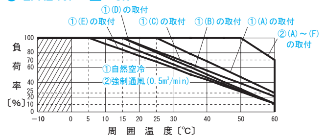
図3.13 動作周囲温度によるディレーティング (参考値)
