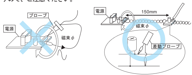
図1.2 出力リップル・リップルノイズ測定例
