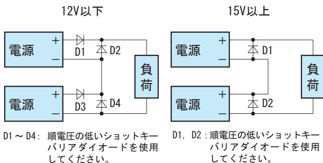
図2.1 直列運転例 (a)
