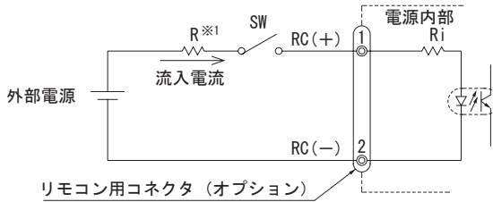
図6.2 リモートコントロール使用例
