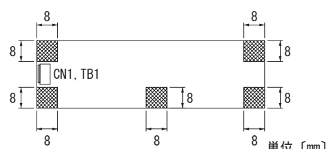
図3.21 取付箇所
