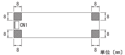
図3.20 取付箇所
