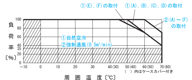
図3.4 動作周囲温度によるデレーティング（参考値）
