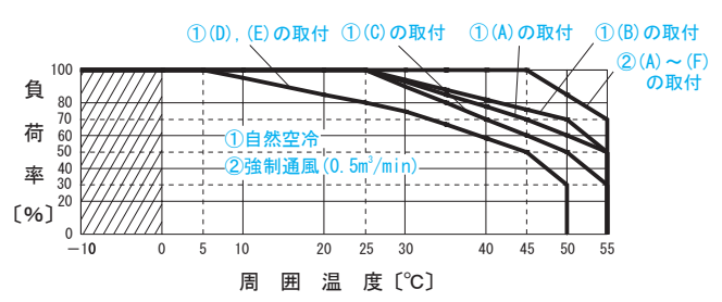
図3.11 動作周囲温度によるディレーティング (参考値)
