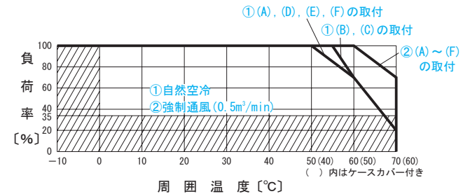
図3.3 動作周囲温度によるデレーティング（参考値）
