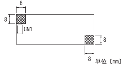
図3.19 取付箇所
