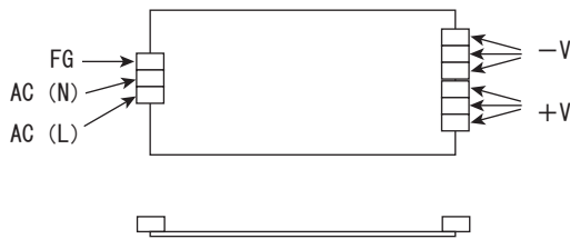
図5.5 -T1端子配列
