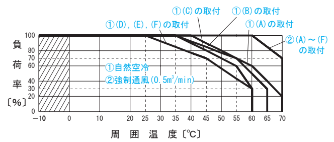
図3.10 動作周囲温度によるディレーティング (参考値)
