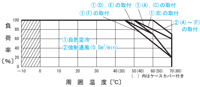
図3.5 動作周囲温度によるディレーティング (参考値)
