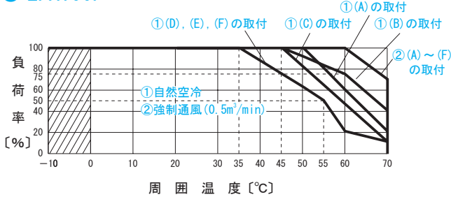
図3.8 動作周囲温度によるディレーティング (参考値)
