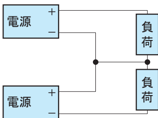
図2.2 直列運転例 (b)
