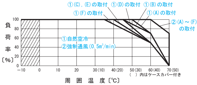
図3.6 動作周囲温度によるディレーティング (参考値)
