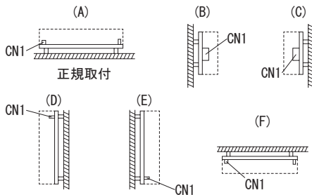
図3.18 取付方法
