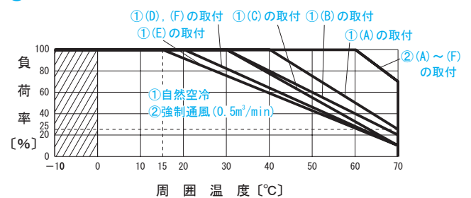
図3.12 動作周囲温度によるディレーティング (参考値)
