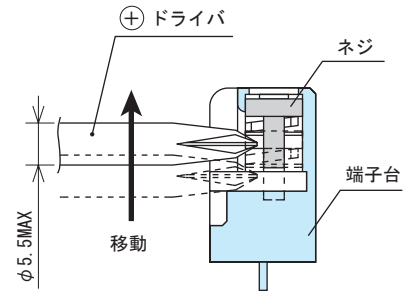
図6.4 ネジ持ち上げ方法
