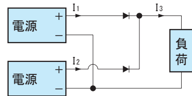
図2.4 冗長運転例
