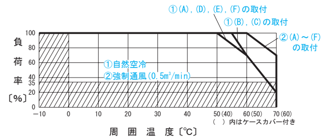
図3.3 動作周囲温度によるデレーティング（参考値）
