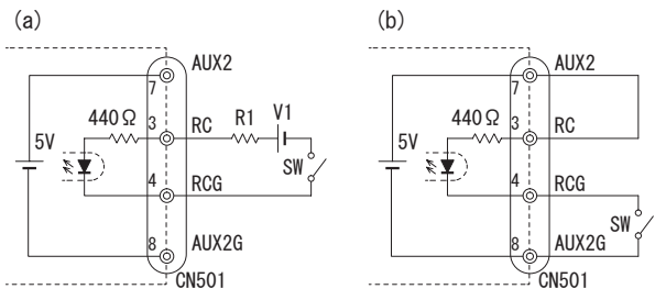
(例 V1:5V R1:270Ω)
