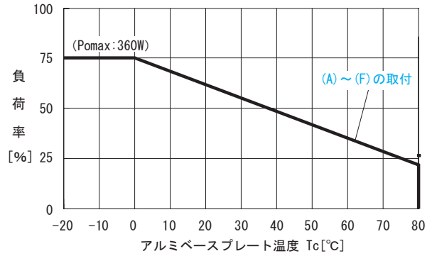
図3.3 伝導冷却におけるベースプレート温度ディレーティング（参考値）
