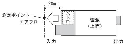
図6.6 ファン排気温度測定ポイント
