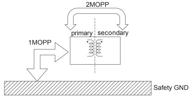
図 6.8 医用規格絶縁クラス
