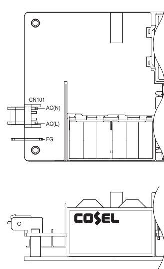
図6.1 -J3仕様の例
