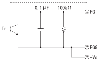
図 6.2 PG 信号の内部回路
