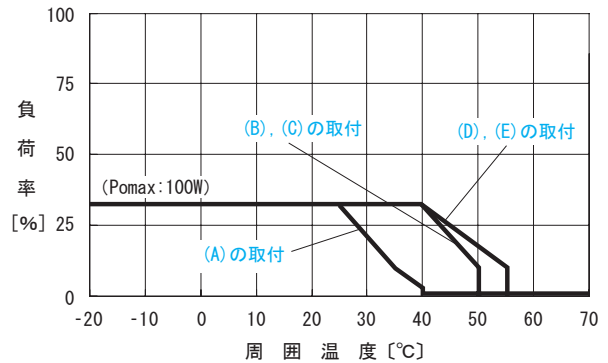
図3.5 自然空冷における動作周囲温度ディレーティング（参考値）
