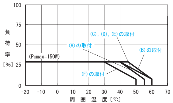
図3.4 自然空冷における動作周囲温度ディレーティング（参考値）
