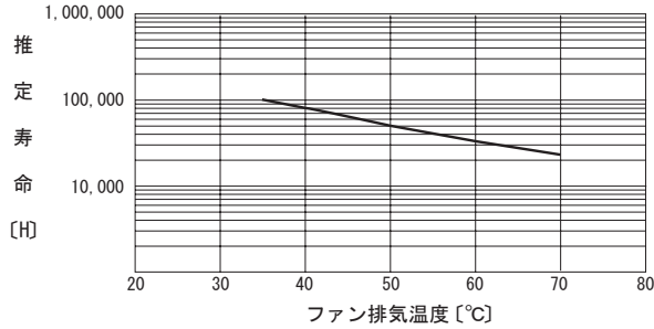
図6.5 ファン推定寿命
