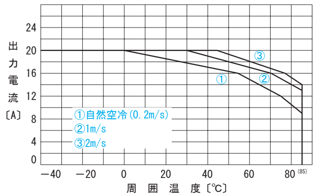
図8.19 CES48050-20P 周囲温度ディレーティング (Vin=48V)
