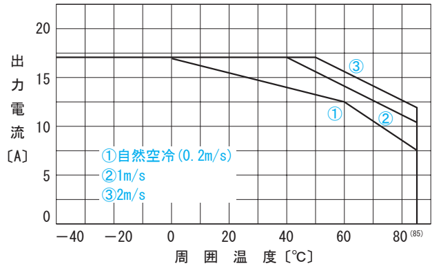
図8.17 CES48060-17 周囲温度ディレーティング (Vin=48V)
