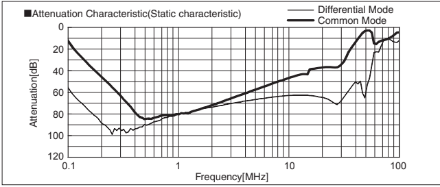
FSB-40-324-U
