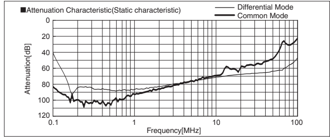
FSB-20-104
