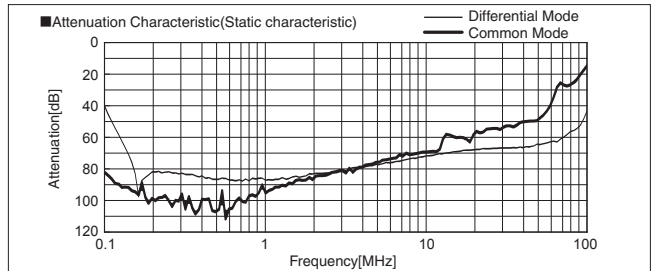
FSB-30-104
