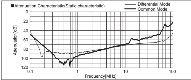
FSB-20-693
