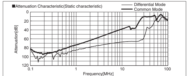
FSB-150-104-U
