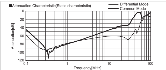
FSB-60-693-U
