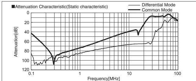
FSB-150-693-U
