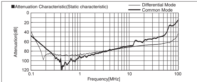
FSB-30-693
