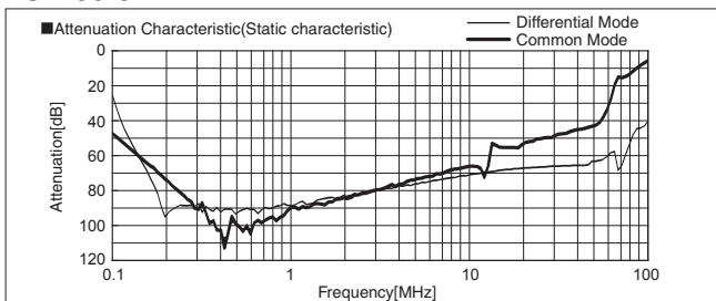
FSB-30-324
