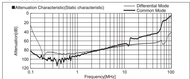
FSB-30-355
