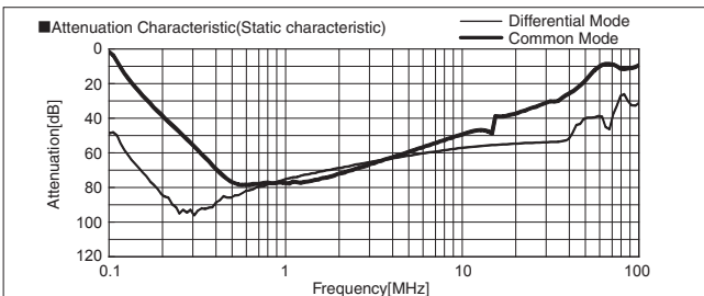
FSB-60-324-U
