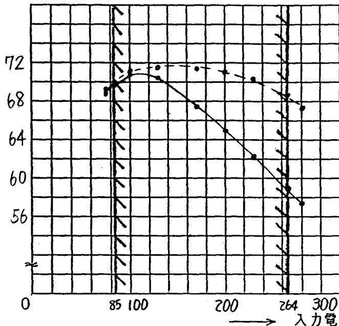
1. グラフ 効率(%)
