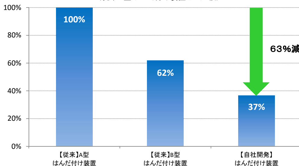
従来はんだ槽との電力使用量比率 (従来A型はんだ付け装置との比較)
