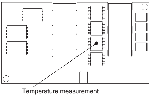
Fig.8.18 CQS48015-50, CQS48018-50, CQS48025-45, CQS48033-45, Temperature measurement location
