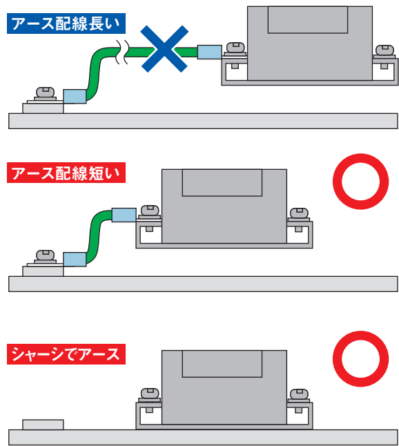
図 3.1.2 アース配線の違い
