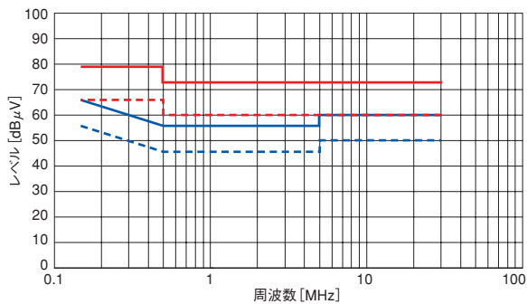
— EN55011 ClassB QP (グループ1) - - EN55011 ClassB AV (グループ1) — EN55011 ClassA QP (グループ1) - - EN55011 ClassA AV (グループ1) (EN55013、EN55014-1、EN55022、EN60601-1も同様)
