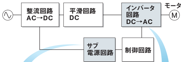
図 1.2.2 汎用インバータブロック図
