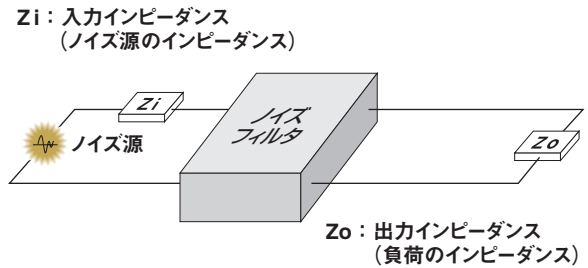
図 4.1.1 フィルタ回路の入出カインピーダンス
