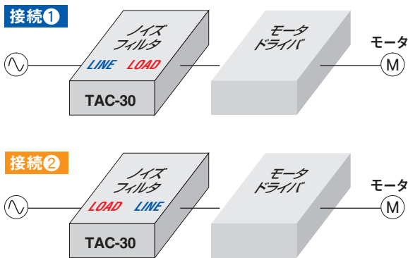
図 4.2.1 ノイズフィルタ取り付け接続方向
