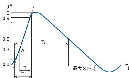
図 5.8.1 電圧サージ波形の例
