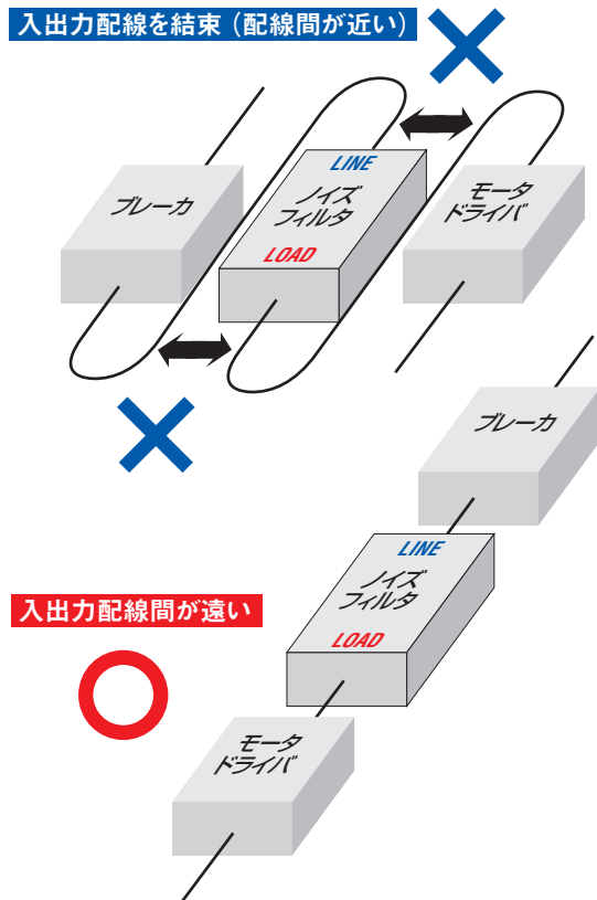
図 3.2.2 入出力配線
