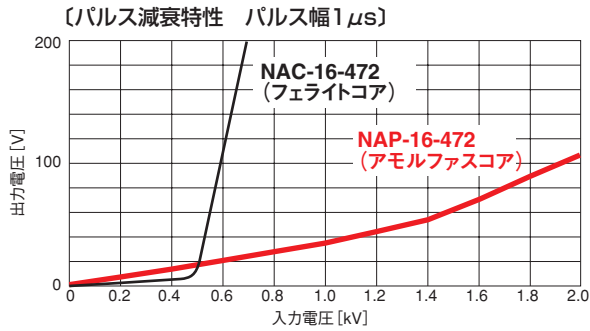
図 2.11.2 パルス減衰特性の比較例
