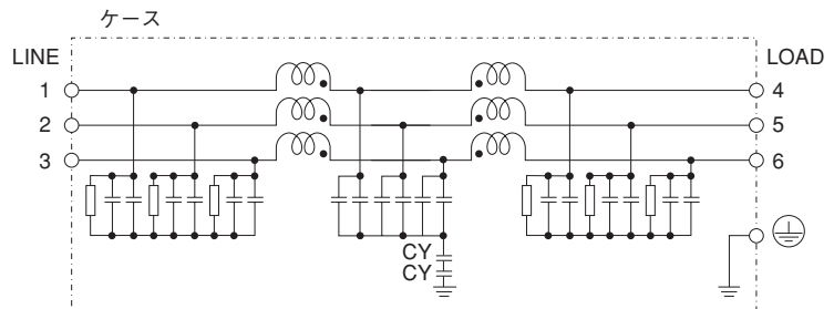
図 4.2.4 TBC シリーズ回路図 (回路が対称)
