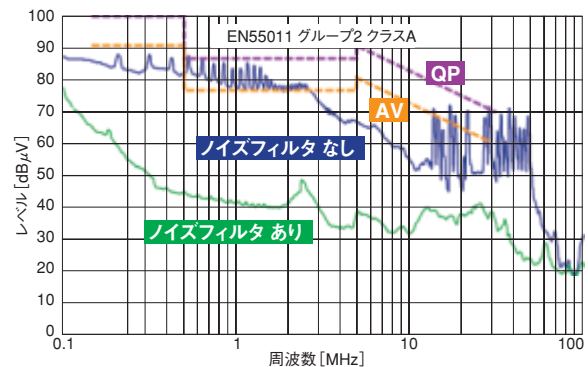
図 1.7.1 ノイズフィルタによる雑音端子電圧低減効果例
