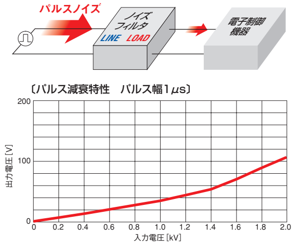
図 1.7.3 パルス減衰特性の例 (NAP-16-472)
