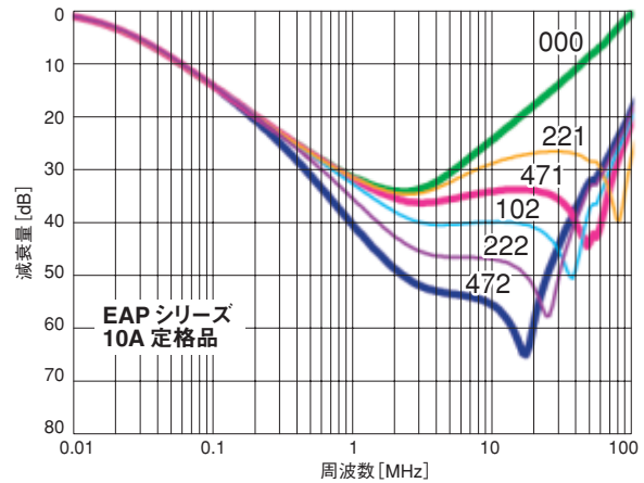
図 2.12.1 接地コンデンサコードとコモン減衰特性例
