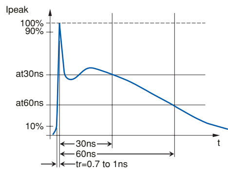
図 5.5.1 放電電流波形
