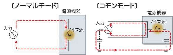
図 1.6.1 ノイズ発生経路 (電源機器内部にノイズ発生源がある場合の例)
