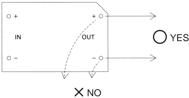
Fig.5.1 Pattern wiring
