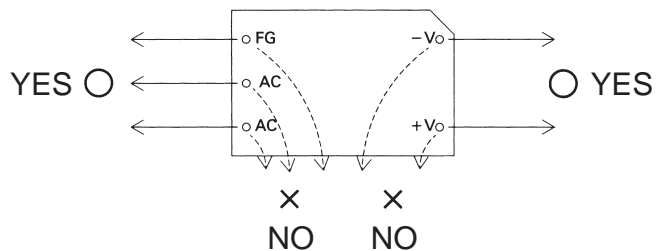
Fig.5.1 Pattern wiring
