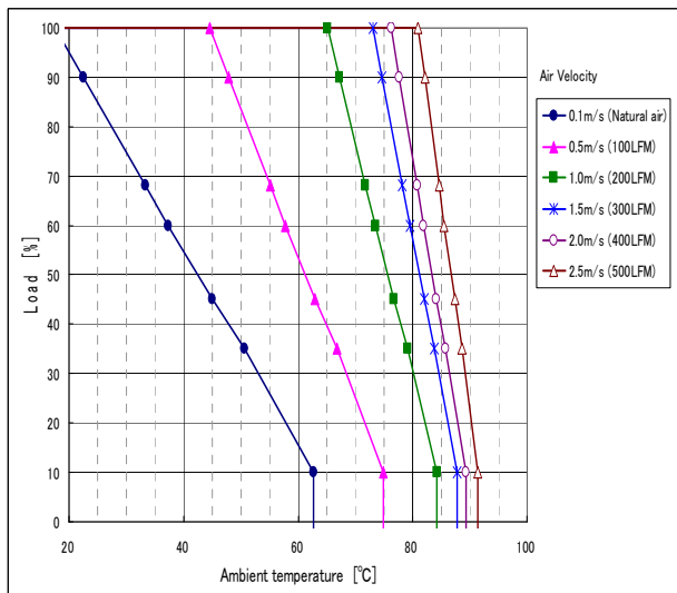
F-QB-F5/F6 (H = 25.4mm)
