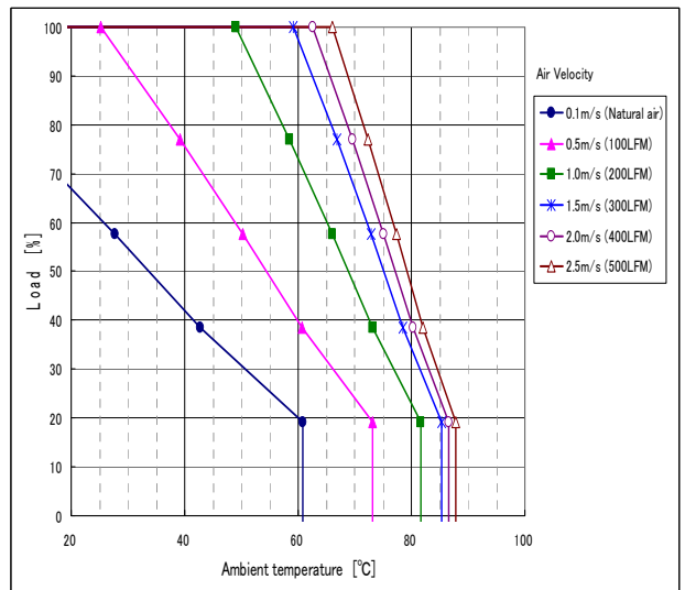
F-CBS-F5/F6 (H = 25.4mm)
