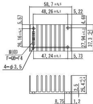
図5 F-QB-F4の外形図
