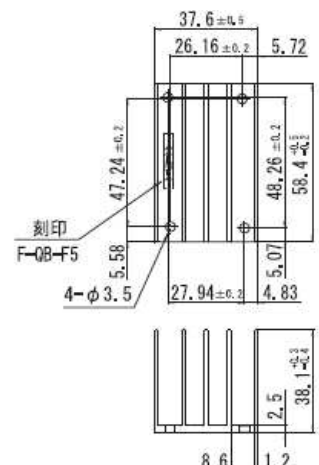
図3 F-QB-F5の外形図
