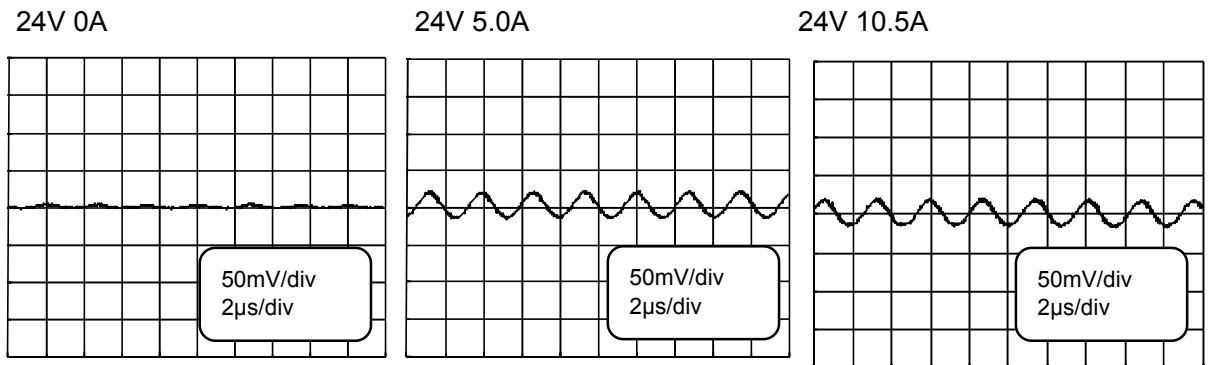
Fig. 10.10 Output noise
