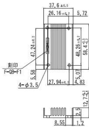
図1 F-QB-F1の外形図
