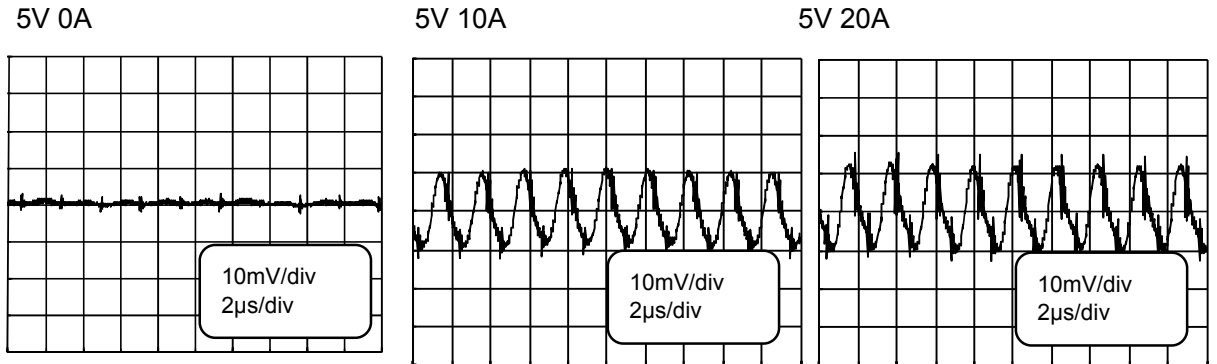
Fig. 10.8 Output noise
