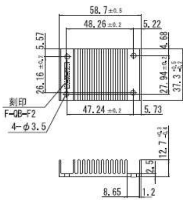
図4 F-QB-F2の外形図
