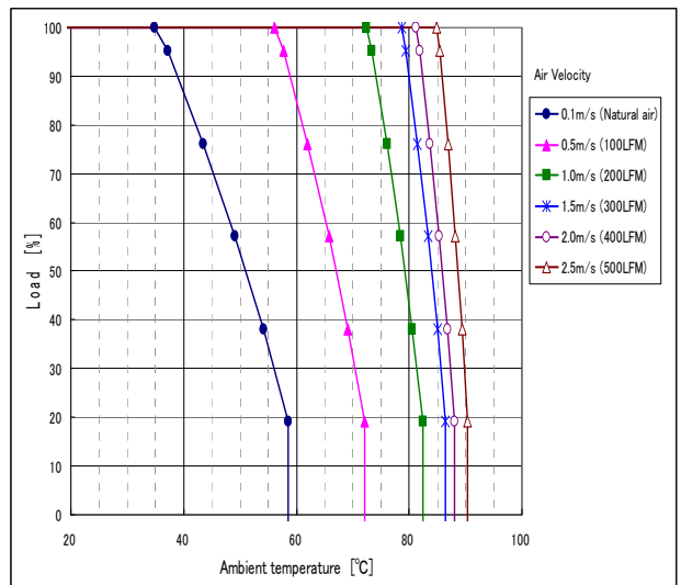
F-QB-F5/F6 (H = 25.4mm)
