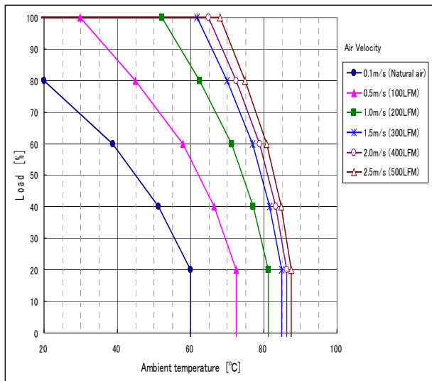
F-CBS-F5/F6 (H = 25.4mm)
