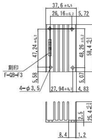
図2 F-QB-F3の外形図
