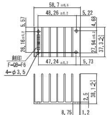
図6 F-QB-F6の外形図
